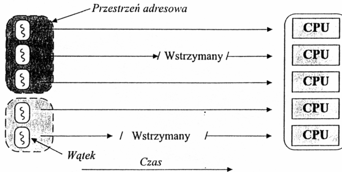
Rysunek 3-3. Procesy wielowątkowe w wieloprocesorze
