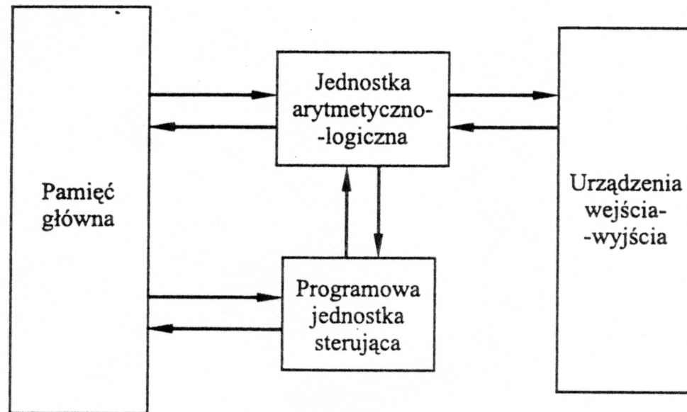
RYSUNEK 2.1. Struktura komputera IAS
