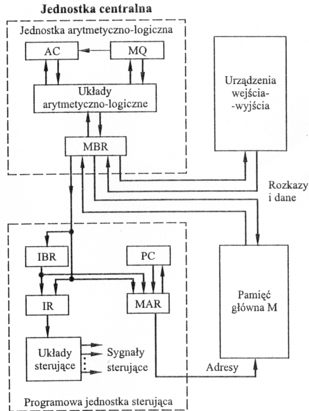
RYSUNEK 2.3. Struktura komputera IAS
