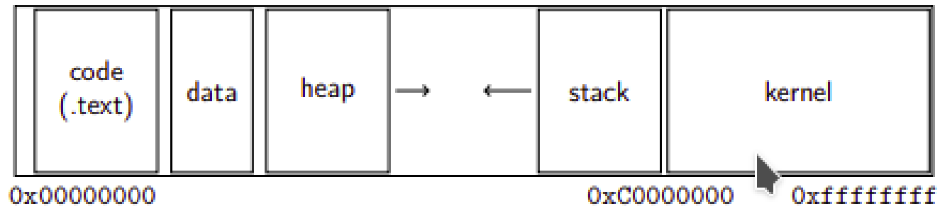
architektura x86
