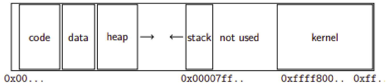
architektura x86_64
